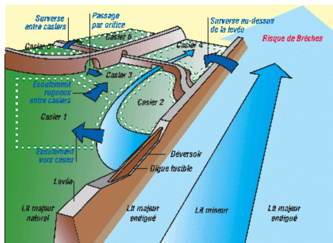
Figure 17 : Représentation d'un modèle à casier
