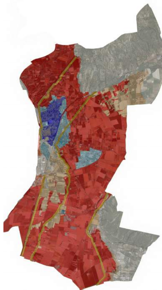
Figure 24 : Type de zonage règlementaire après qualification RAR du système de protection rive gauche de la digue de la Montagnette à la digue Ouest au remblai ferroviaire et révision du PPRi : le zonage bleu clair « évolution après qualification du système » figurant ci-dessus de manière indicative sera défini précisément dans le cadre de la révision du PPRi sur la base notamment du dossier de qualification délimitant la zone protégée (Annexe 5 : Carte des possibilités d'évolution du zonage règlementaire après qualification du système de protection)
