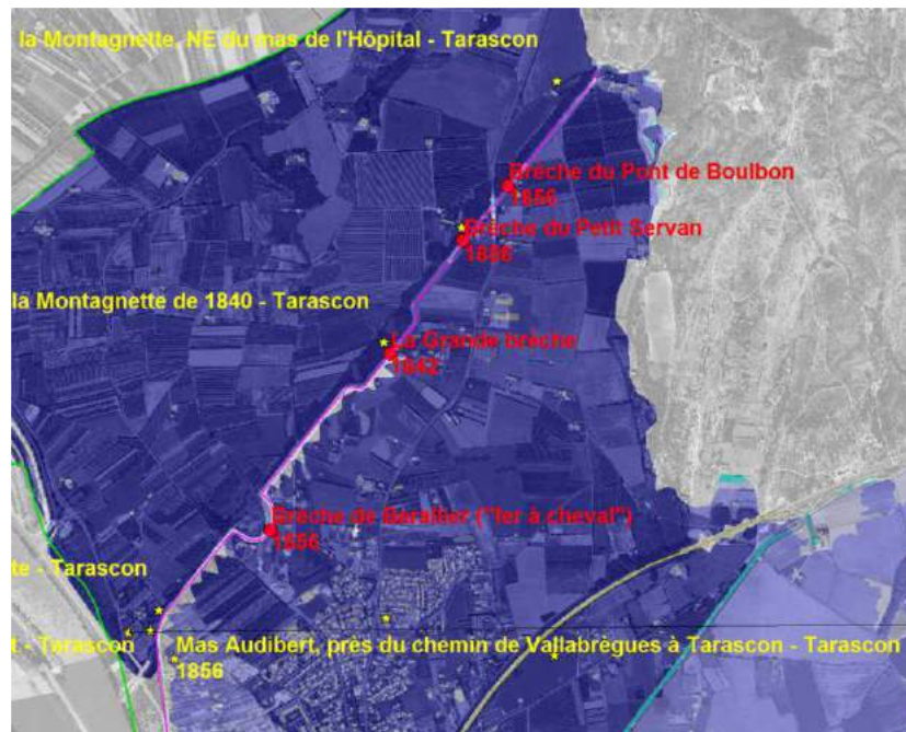
Figure 12 : Brèches historiques dans la digue de la Montagnette
