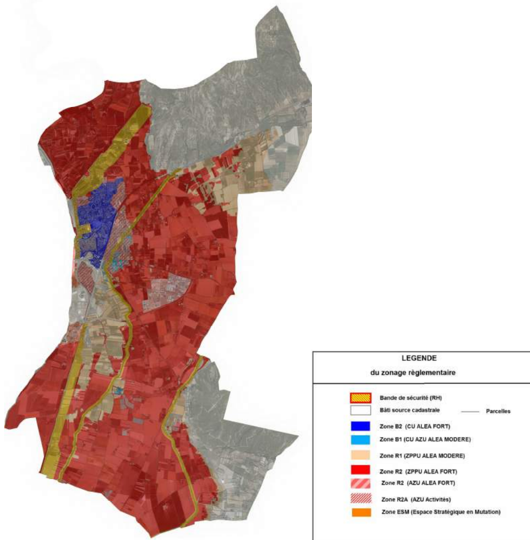
Figure 23 : Zonage réglementaire du présent PPRi (Pièce 2a : zonage réglementaire sur l'ensemble du territoire communal Echelle : 11 000 e )
